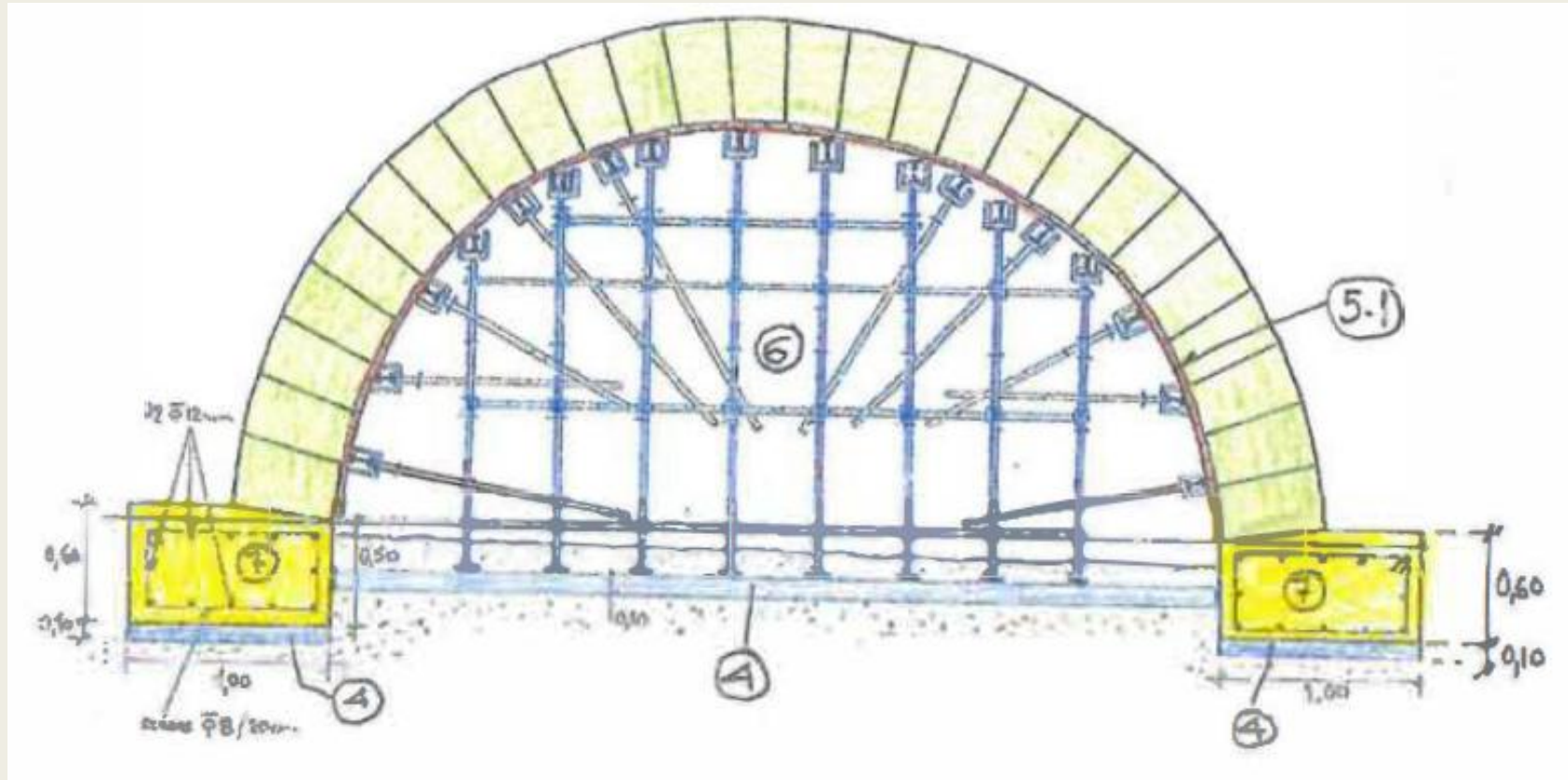
Arco nº 15 – 2ª fase de reparación
